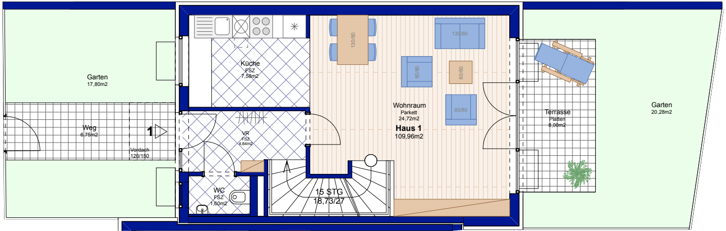
Erdgeschoss
